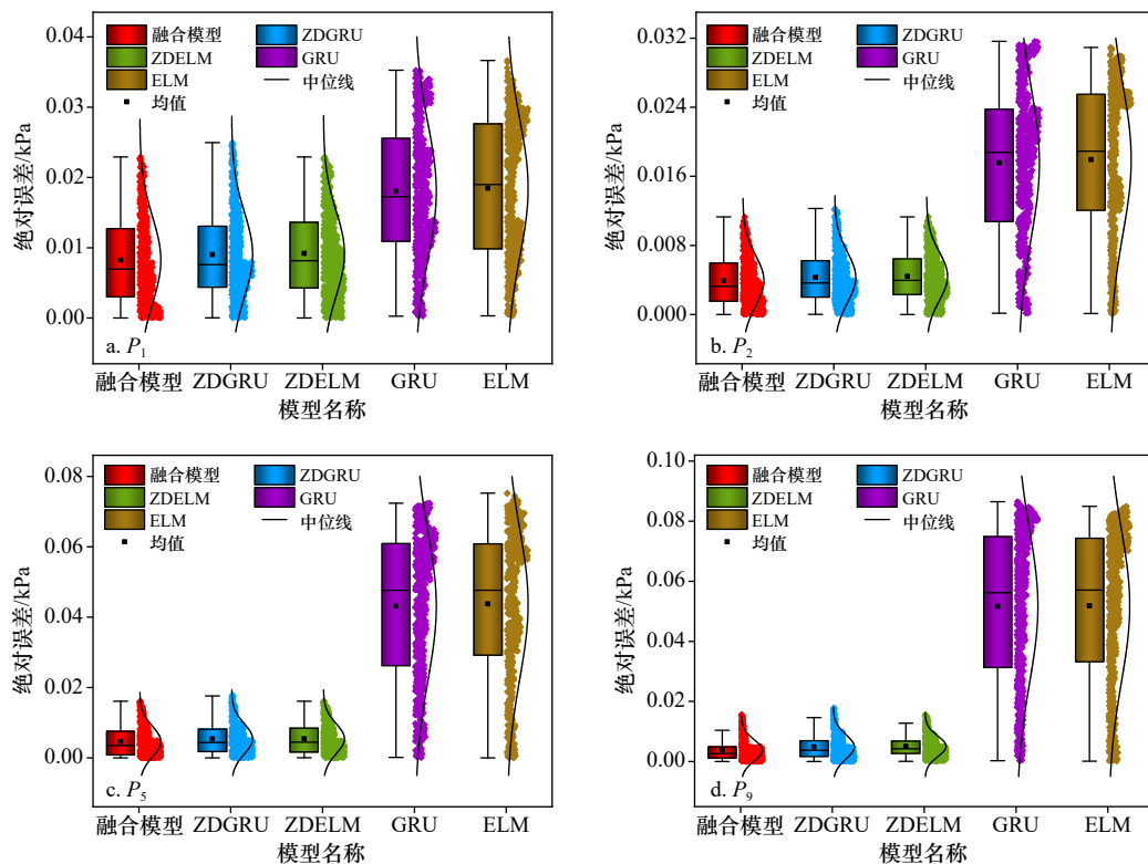
图 12 绝对误差箱型分布
