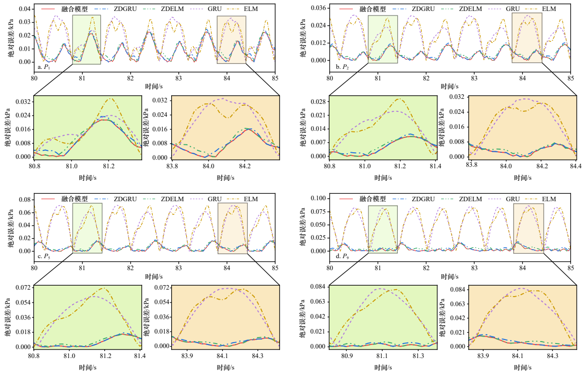
图 11 绝对误差演变曲线
