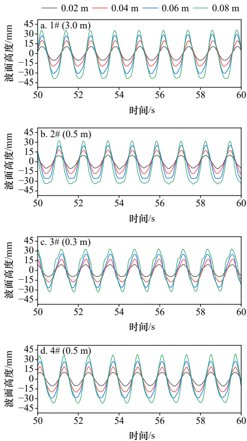
图5 不同波高面历时曲线
