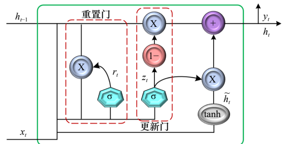
$x_i$ 为输入; $y_i$ 为输出; $r_i$ 为重置门; $z_i$ 为更新门; $h_i$ 为最终隐藏状态; $\sigma$ 为 sigmoid 函数; $\tilde{h}_i$ 为候选隐藏状态
