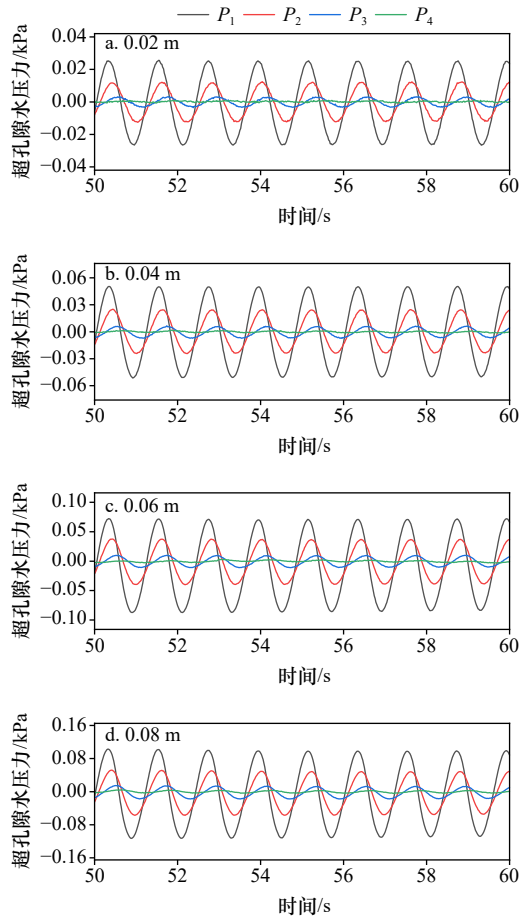
图6 前侧超孔隙水压力历时曲线
