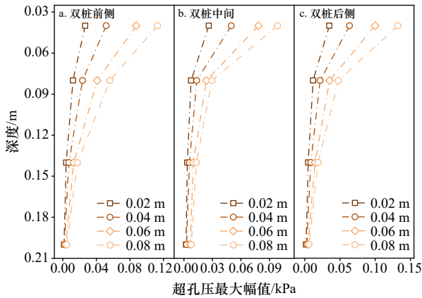
图 7 超孔压最大幅值对比
