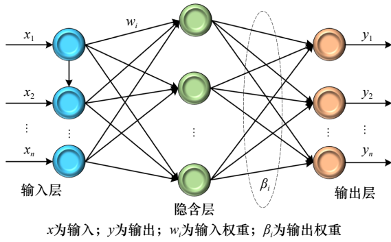
图4 ELM网络结构
