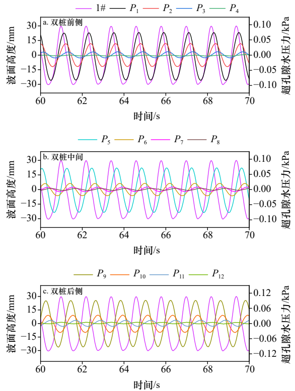
图 8 实际波高与超孔压(入射波高 0.06 m 工况下)
