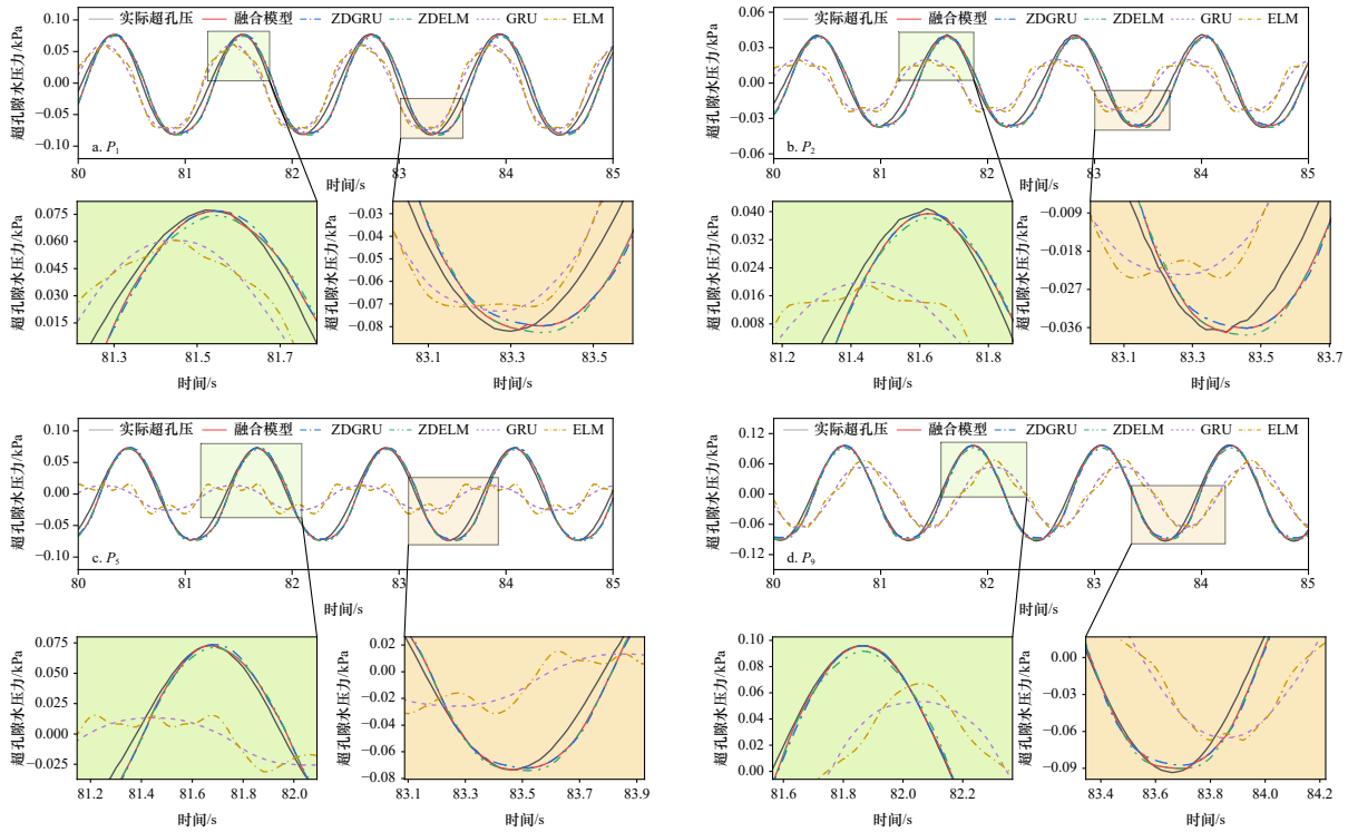
图 14 超孔压幅值预测结果
